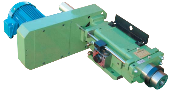
馬達盒組合
